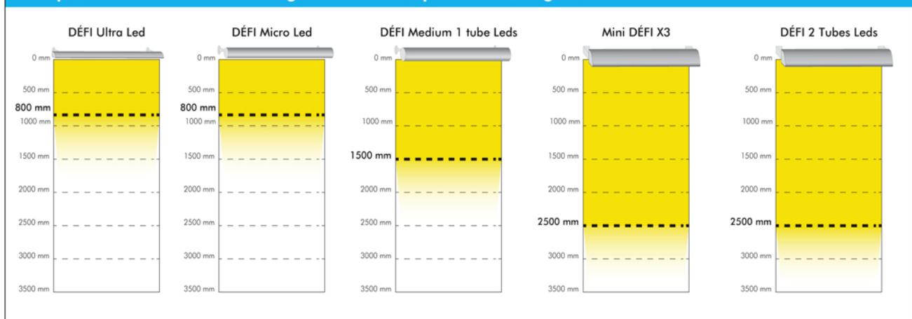
Comparatif de la hauteur d'éclairage en fonction du profilé d'éclairage Leds choisi :
