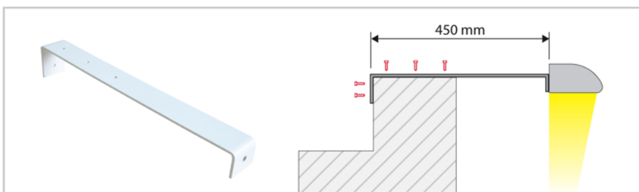
Fixation par acrotère - Lg : 450 mm 4 points de fixation
