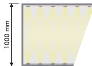
Leds périphériques 3 W
