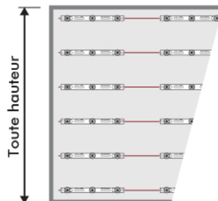
Barres de Leds rasantes étanches
