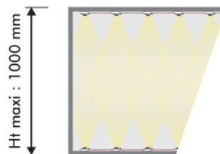
Leds périphériques 3 W
