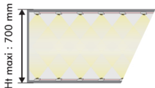
Leds périphériques 1,32 W
