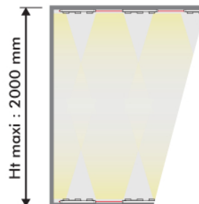
Leds périphériques 3 x 2 W LG - étanches
