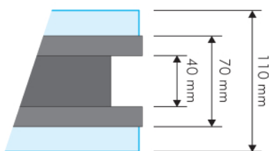
Modules Leds périphériques 3 W
